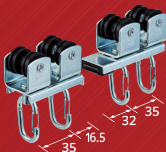
ベンダーマグネットランナー(両開) ワンタッチランナータイプ
