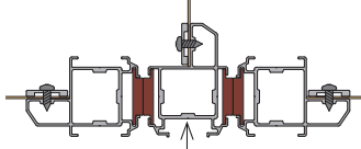
三方納まり図
