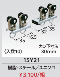
D40マグネットランナー(両開) スチールランナータイプ
