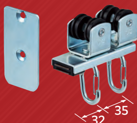
ベンダー片マグネットランナー(片開) ワンタッチランナータイプ
